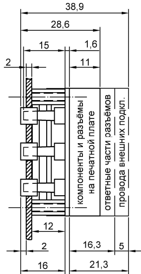
Чертеж для варианта расположения кнопок справа от дисплея
