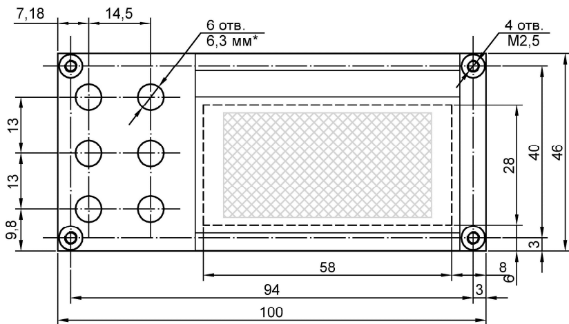
Чертеж для варианта расположения кнопок слева от дисплея
