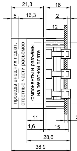
Чертеж для варианта расположения кнопок слева от дисплея
