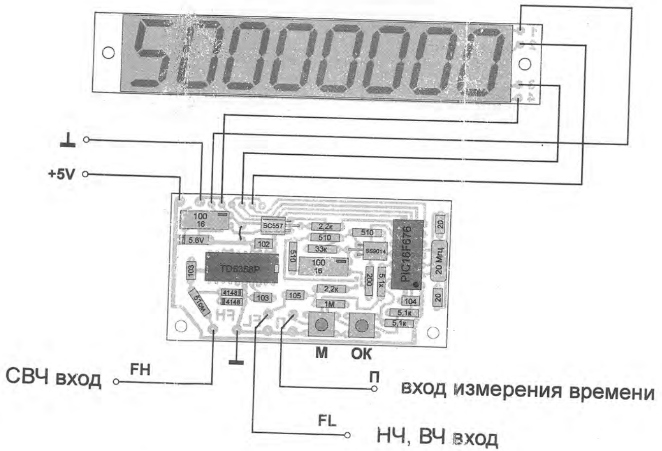
Рис.2 Схема монтажа частотомера.
