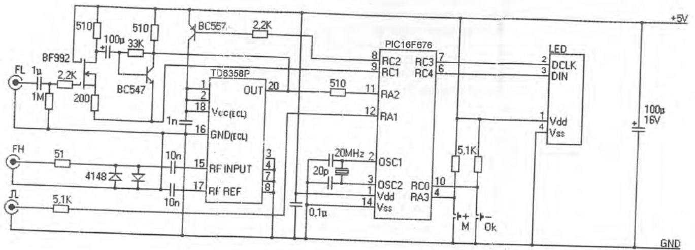
Рис.1 Принципиальная схема частотомера.
