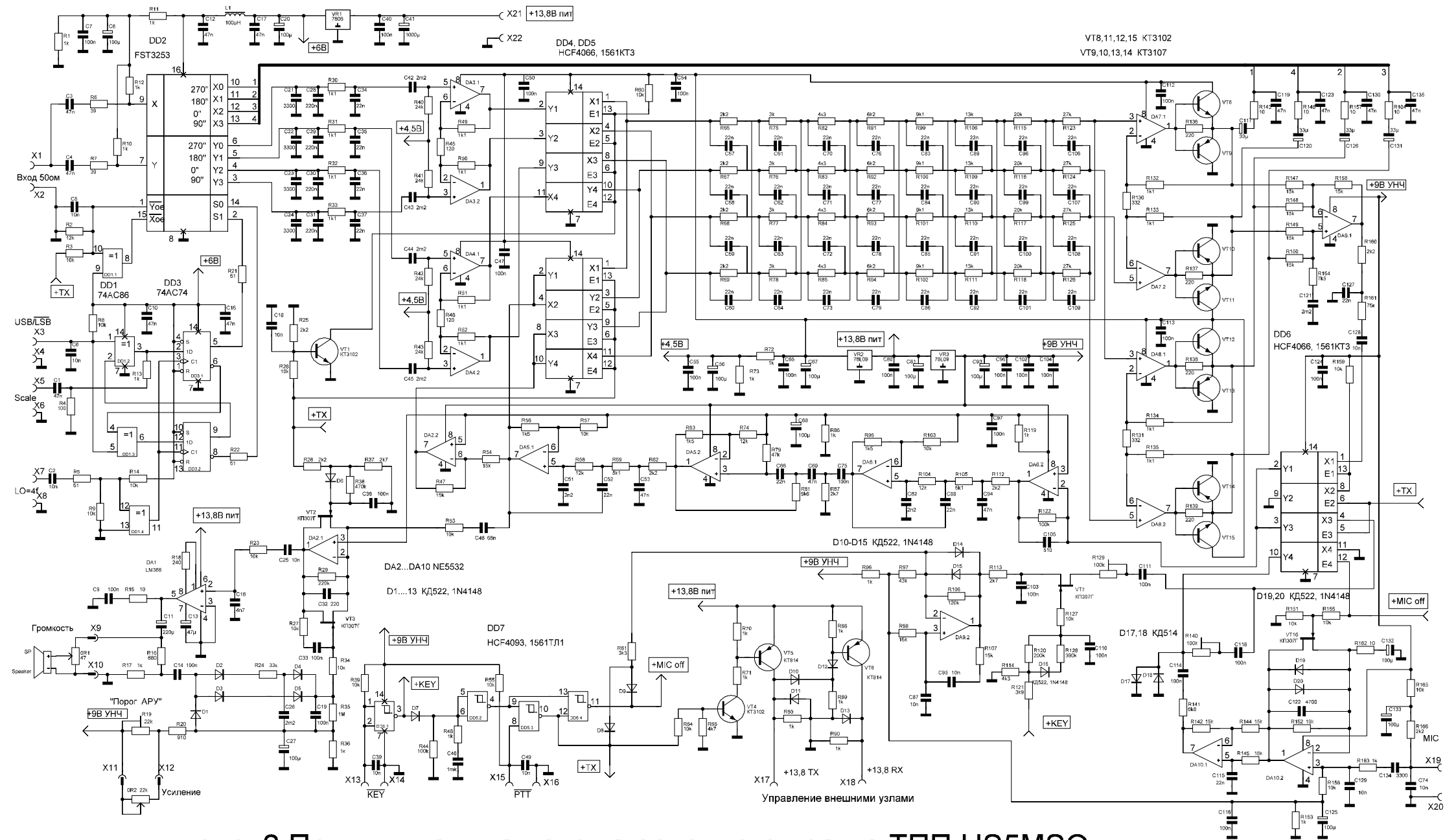
рис. 2 Принципиальная схема основного тракта ТПП US5MSQ
