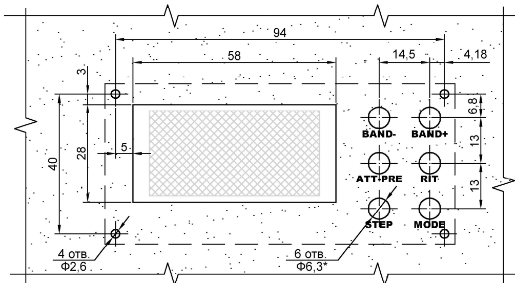
Фрагмент фальшпанели с разметкой отверстий для установки синтезатора
