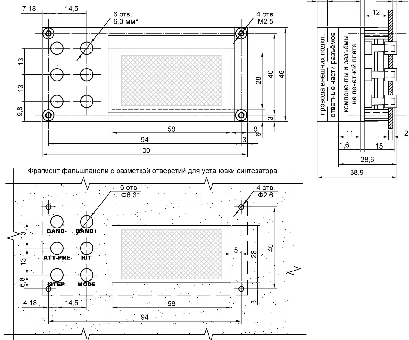
Чертёж для варианта расположения кнопок слева от дисплея
