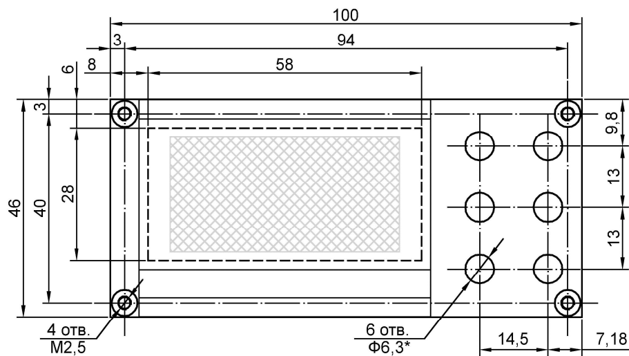
Фрагмент фальшпанели с разметкой отверстий для установки синтезатора
